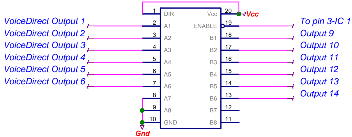
IC 4 74LS245
